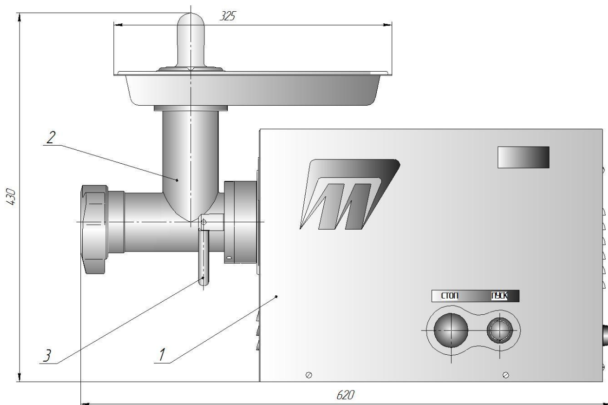
Рисунок 1 – Мясорубка М-80М/220
