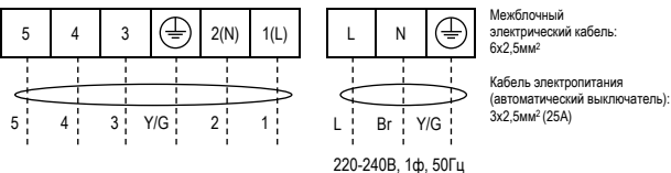
Внутренний блок модели ASW-H24A4/FP-R1
