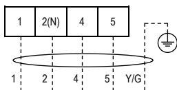
Наружные блоки моделей AS-H07,09,12,18A4/FP-R1
