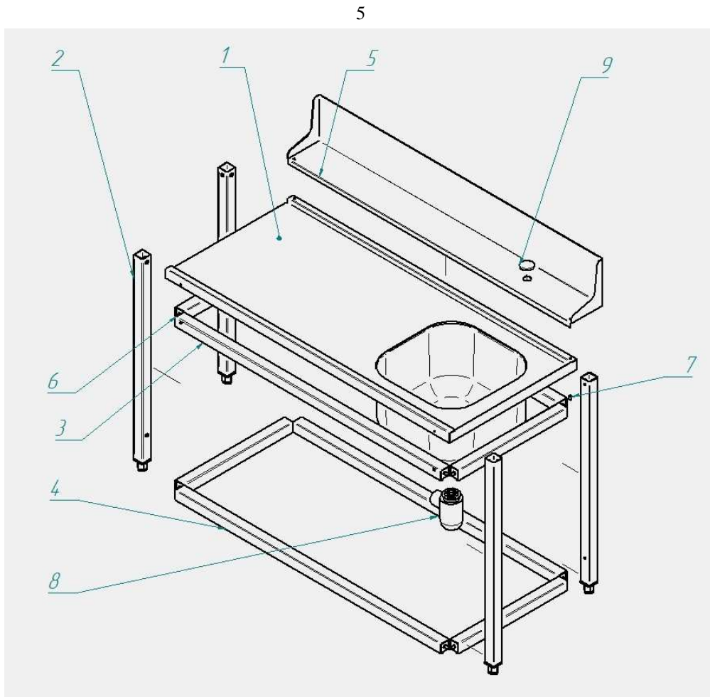
Рис. 1 Разнесенная сборка стола предмоечного СМПП-7-4
