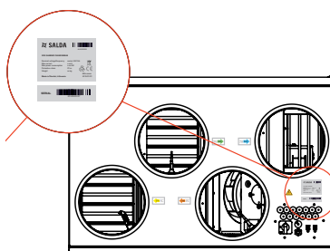
Рис. 2.2. Место технической этикетки на RIS V EKO 3.0
