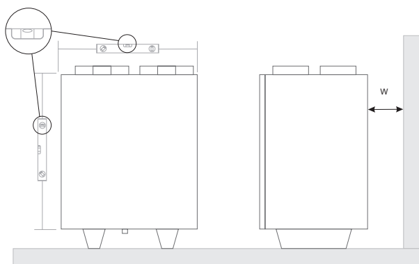
Рис. 13.1. RIS 700 V ЕКО 3.0 позиция монтажа ( W=400 \text{ mm} )
