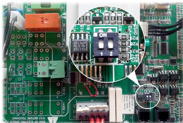
Рис. 19.2.3. Микровыключатели 1 и 2
