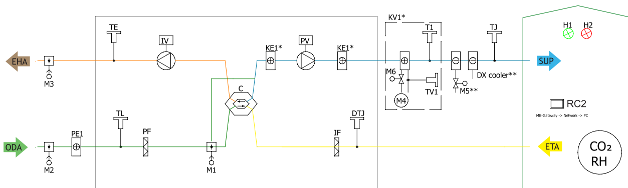
Рис. 15.1. RIS 700 V EKO 3.0 (* KE1 – используется в электрической версии. В горизонтальной версии нагреватель находится перед приточным вентилятором; * KV1 - используется в водяной версии. Для большей информации, читайте инструкцию. ** Возможно контролировать. PE1 – саморегулирующийся предварительный нагреватель)
