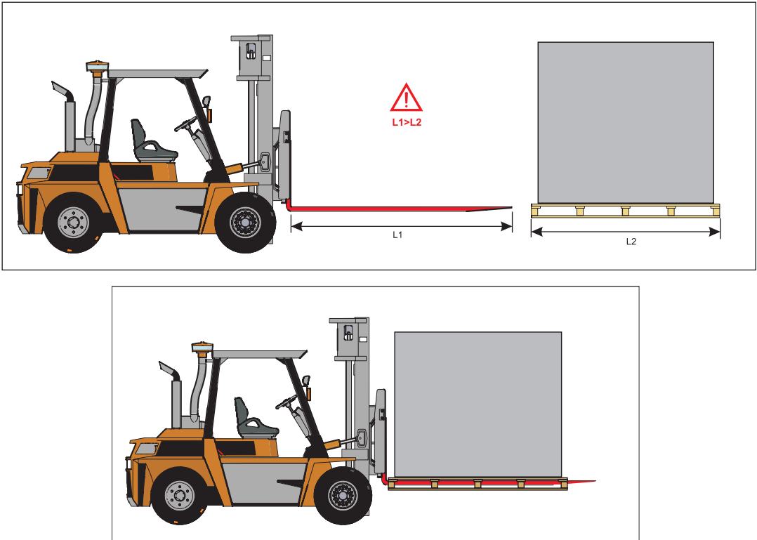
Рис. 9.1. Подъем грузоподъемником
