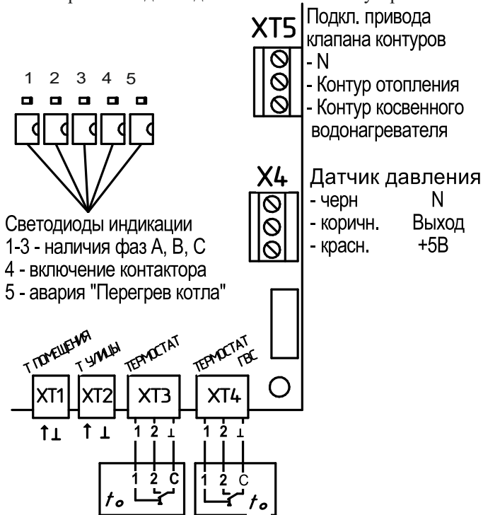
Рисунок 5. Подключение к разъёмам на плате.
