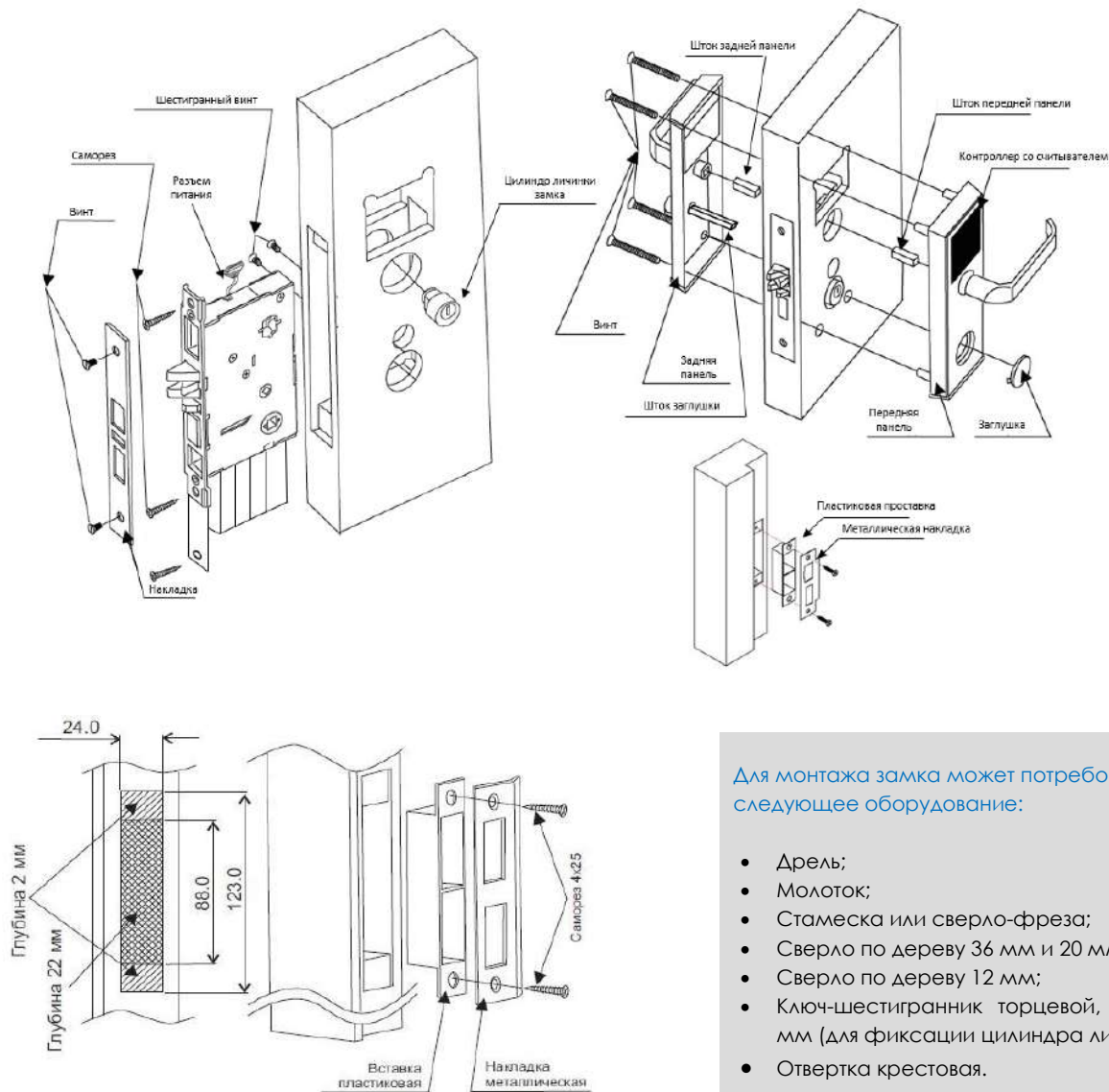
Схема монтажа
