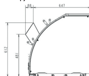
Лоток подачи для ручной загрузки
