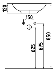
HARMONY РАКОВИНА НА СТОЛЕШНИЦУ HRLG04501FD0W3000 Ø450
