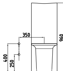
ЛОТУС НАКЛАДНАЯ ПАНЕЛЬ ДЛЯ БАЧКА - МОНОБЛОК LTRY09601FD0W3000 960x360 мм
