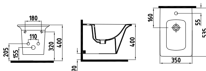
LOTUS ПОДВЕСНОЕ БИДЕ С ГИГИЕНИЧЕСКИМ ПОКРЫТИЕМ (СКРЫТЫЙ МОНТАЖ) С ОТВЕРСТИЕМ ПОД СМЕСИТЕЛЬ LTBA05401VD1W3000 535 x 350 мм
