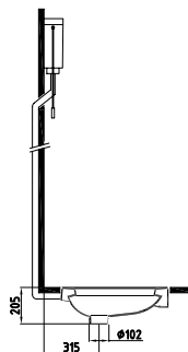
ЧАША ГЕНУЯ TRHT06001VSAW3000 600x600 мм Подвод воды сзади
