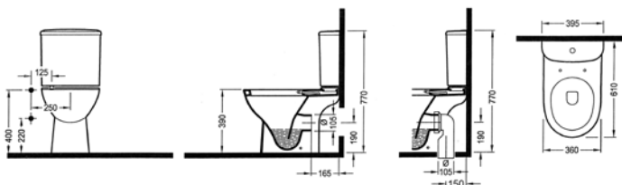
БАЧОК (ПОДВОД ВОДЫ СНИЗУ) TPRS03801VDAW3000 380x395 мм
