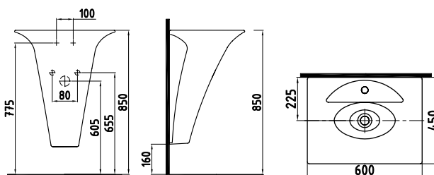
LOTUS ПОДВЕСНАЯ РАКОВИНА МОНОБЛОК LTLM06001FD1W3000 600x450 мм
