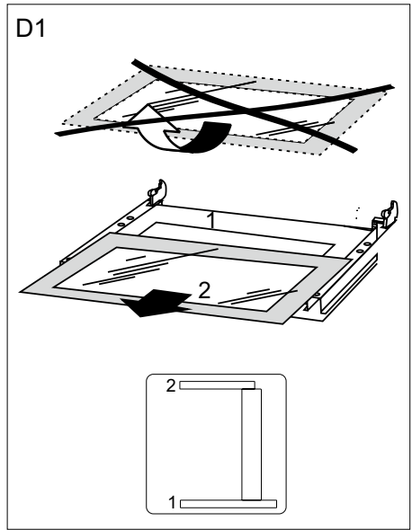
Innenglas entfernen 2 Glas.
