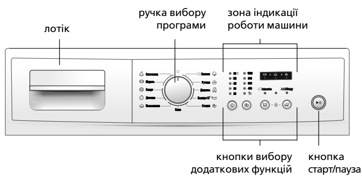
Рисунок 1 – Панель керування
