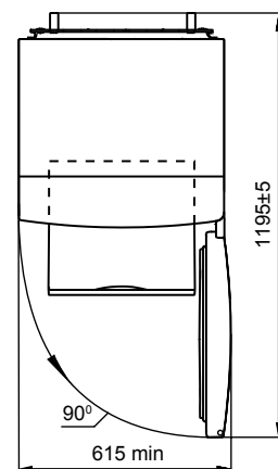
2 сурет – Тоңазытқыш (үстінен қарағанда)
