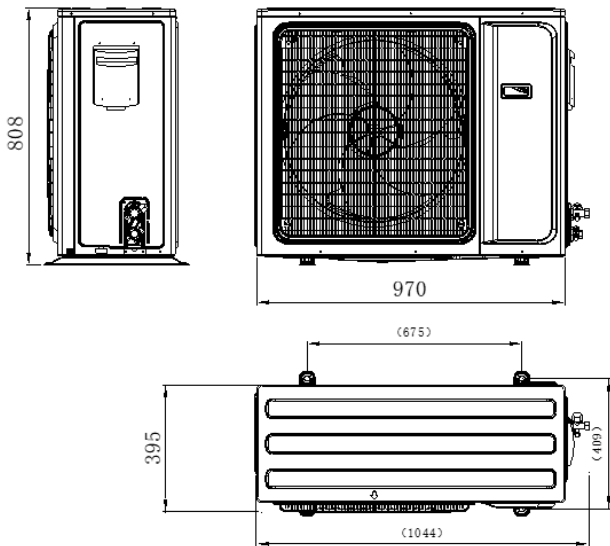
Модель IUX-V36HDC
