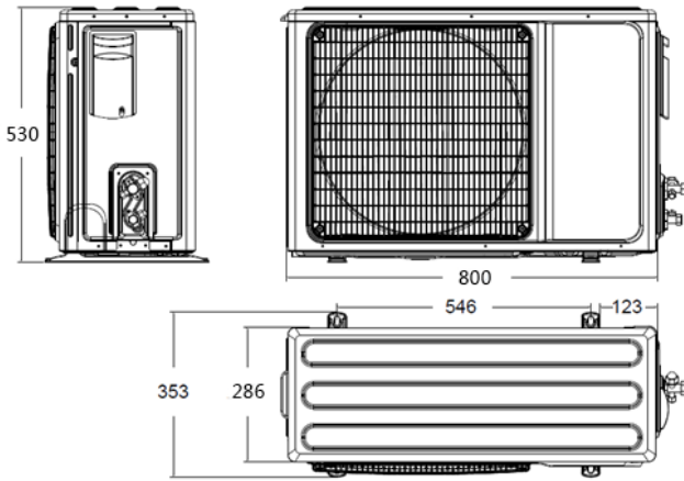
Модель IUX-V18HDC
