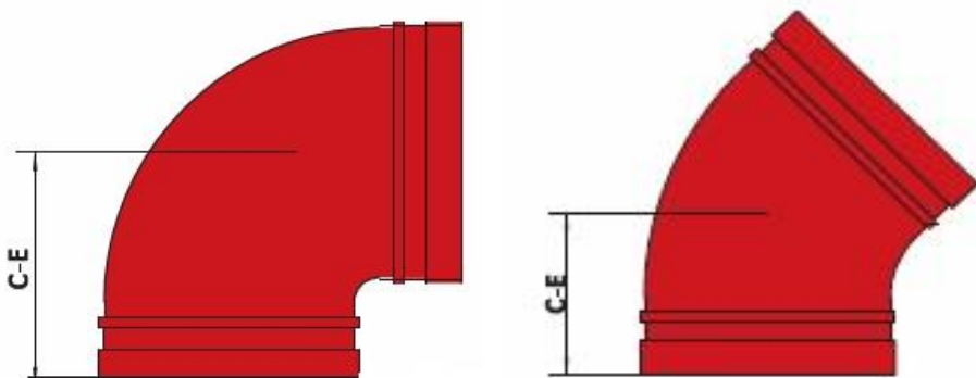
Рис. 1. Размеры отводов «LEDE».
