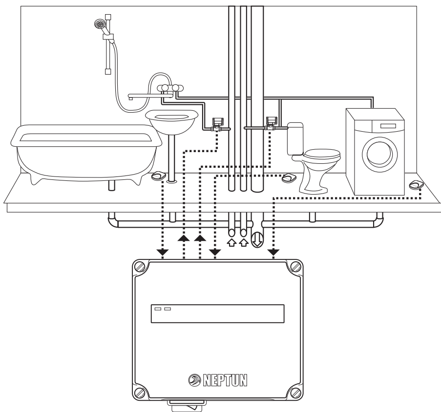
Рис. 1. Пример размещения комплекта в стандартной квартире.
