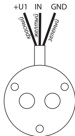
Рис. 5. Маркировка проводов.
