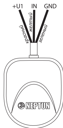
Рис. 7. Маркировка проводов.
