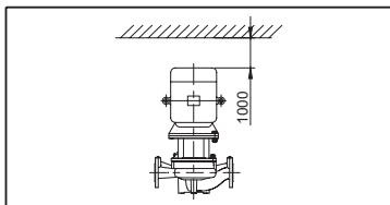
Рис. 8 Расстояния до стен/потолка для насосов TPV
