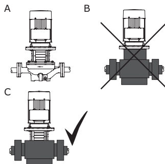
Рис. 12 Изоляция насосов TPV
