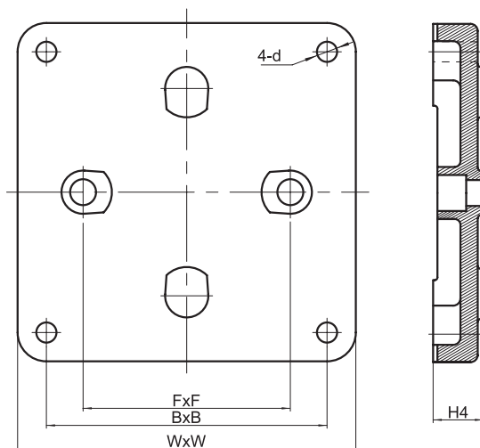
Рис. 19 Примеры и размеры плит-оснований для насосов TPV
