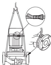
Рис. 4 Насосы TPV без специальных креплений
