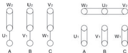
Рис. 17 Схемы подключения \Delta или Y
