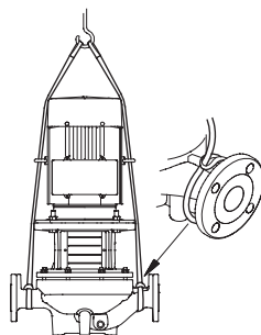
Рис. 5 Насосы TPV со специальными креплениями
