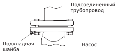
Рис. 6 Использование шайб для овальных отверстий под болты
