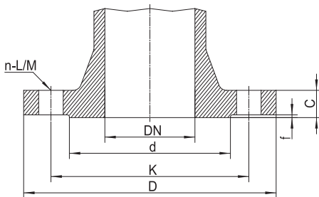
Рис. 18 Характеристики фланцев
