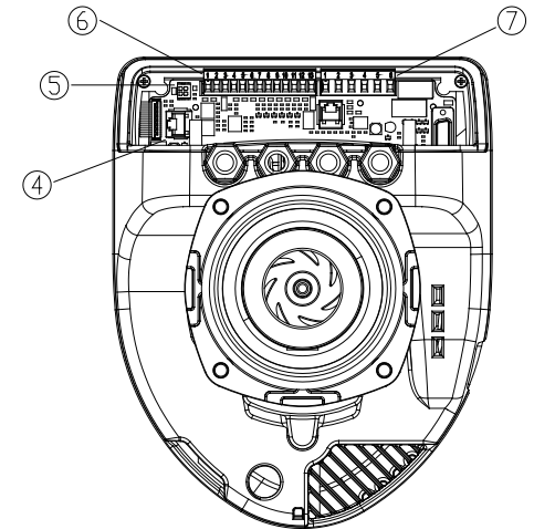
Kuv. 5: Sähköliitännät (taka)
