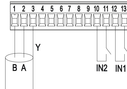
Εικόνα 7: Αφαιρούμενη κλέμμα 13 πόλων: ψηφιακές εισοδοι και MODBUS
