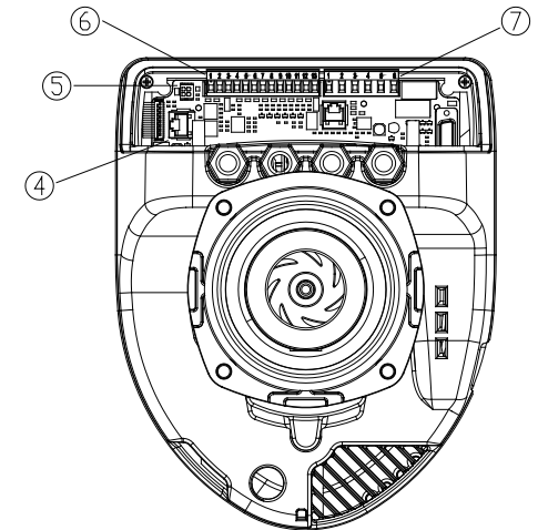
Fig. 5: Elanslutning (baksida)
