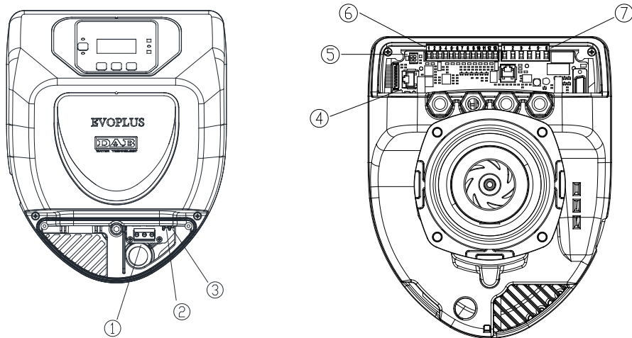
Figure 4 : Connexions électriques (face)
