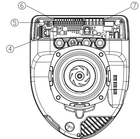
Figura 5: Ligações eléctricas (parte traseira)
