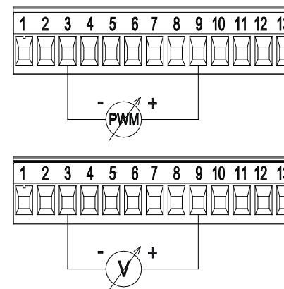
Figura 8: Morsetteria estraibile 13 poli: ingressi 0-10V e PWM
