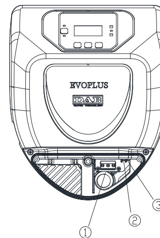
Fig. 4: Elanslutning (framsida)
