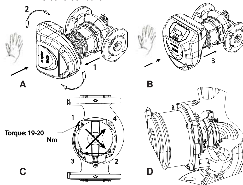
Afbeelding 2: Montage-instructies motorblokken
