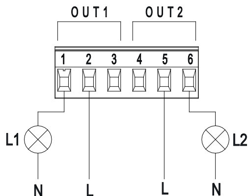
Afbeelding 9: Uittrekbaar 6-polig klemmenbord: aansluitvoorbeeld van de uitgangen
