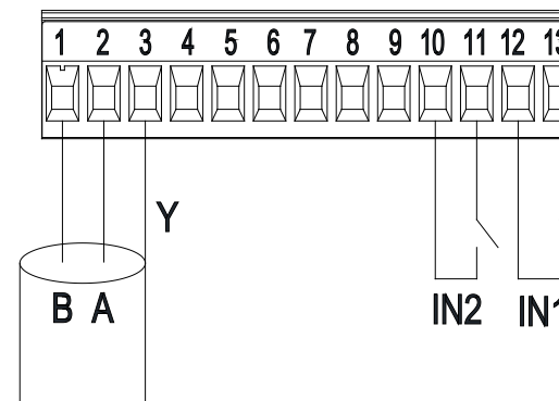
Afbeelding 7: Uittrekbaar 13-polig klemmenbord: digitale ingangen en MODBUS
