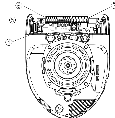
Figura 5: Conexiones eléctricas (parte posterior)
