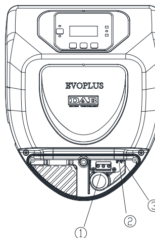
4 pav. Elektros jungtys (priekis)
