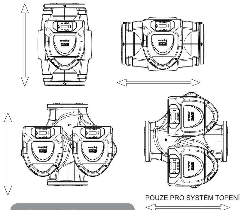
Obr. 1: Poloha montáže
