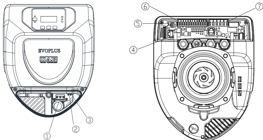
Figura 4: Conexiuni electrice (față)
