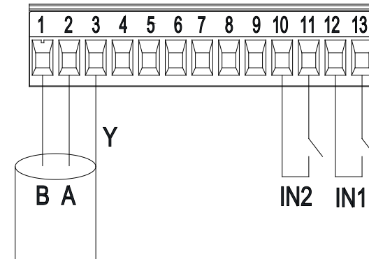
Fig. 7: 13-polig utdragbar kopplingsplint: Digitala ingångar och MODBUS
