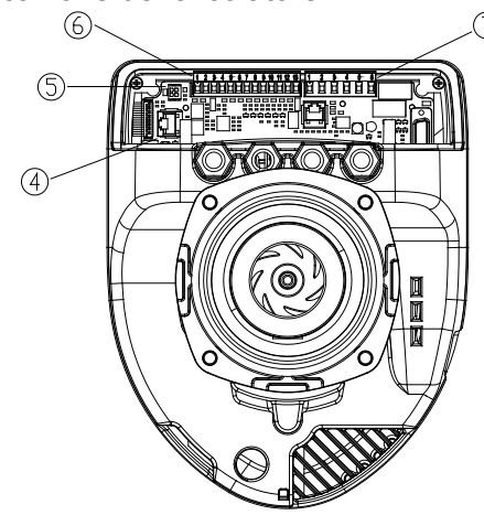
Figura 5: Connessioni elettriche (retro)
