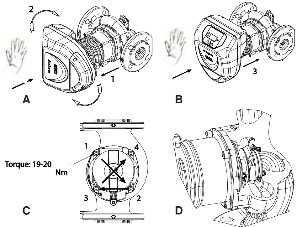
2 pav. Variklio galvučių įrengimo instrukcija
