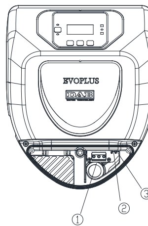
Figura 4: Connessioni elettriche (fronte)
