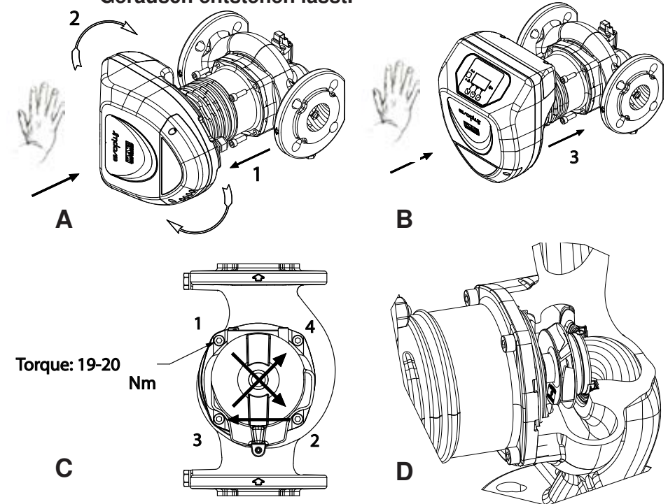
Abbildung 2: Montageanleitungen für Motorkopf
