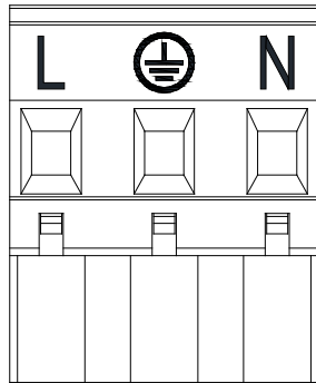
Figura 6: Morsettiera estraibile di alimentazione
