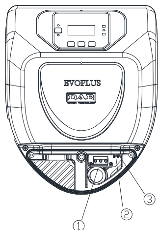
Rys. 4: Podłączenia elektryczne (przód)
