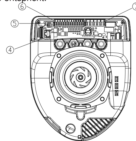
Abbildung 5: Elektroanschlüsse (Rückseite)
