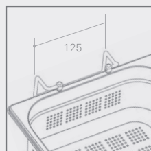
Foratura fondo Perforated bottom h 65
