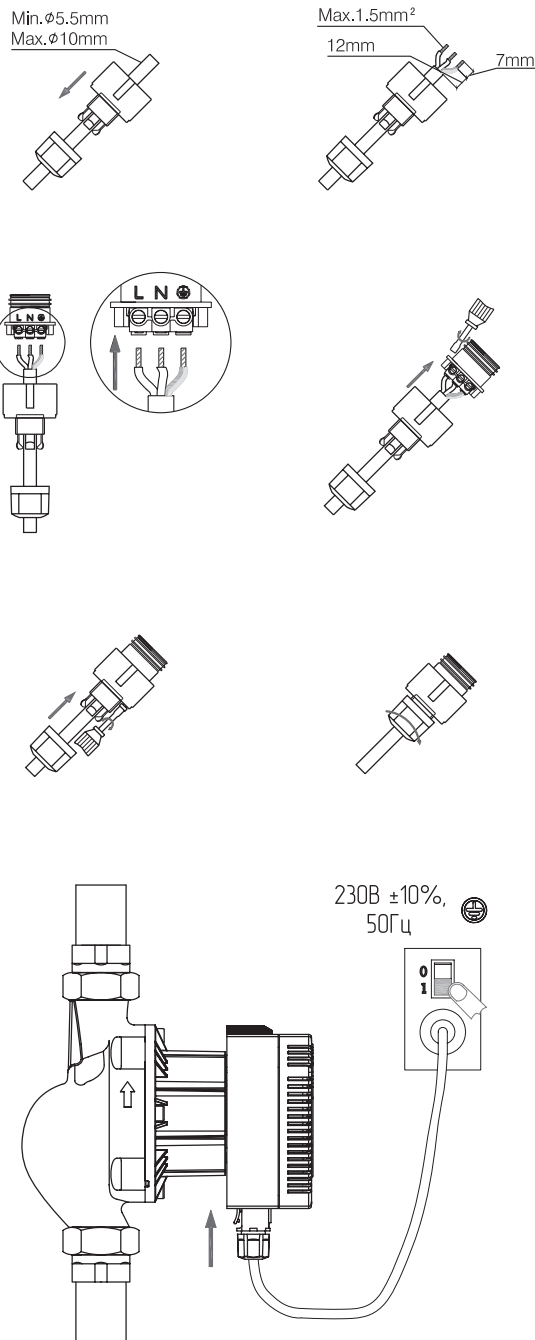
Рис. 36 Электроподключение насоса
