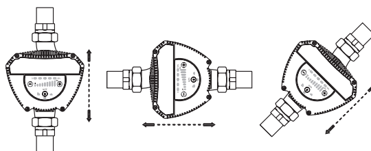
Рис. 33 Допустимое расположение вала насоса
