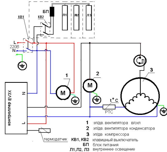
17.1 Электрическая схема стола TN (HT - в исполнении с дополнительным внутренним освещением).
