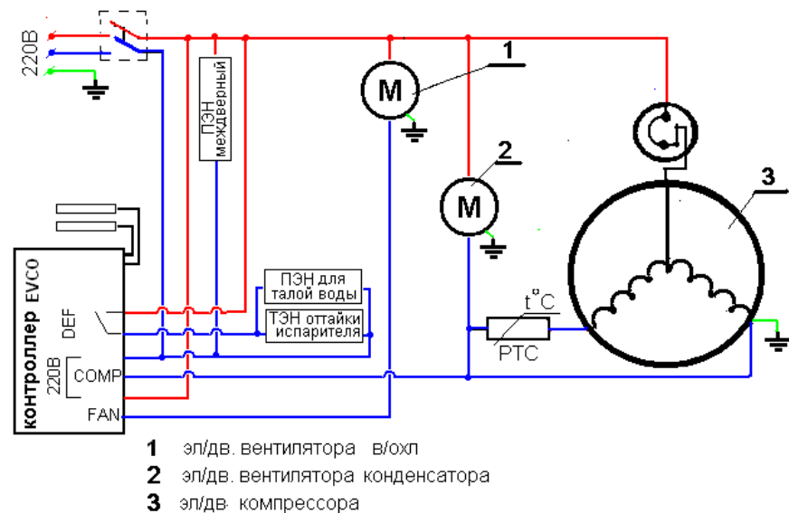
17.2 Электрическая схема стола BT.
