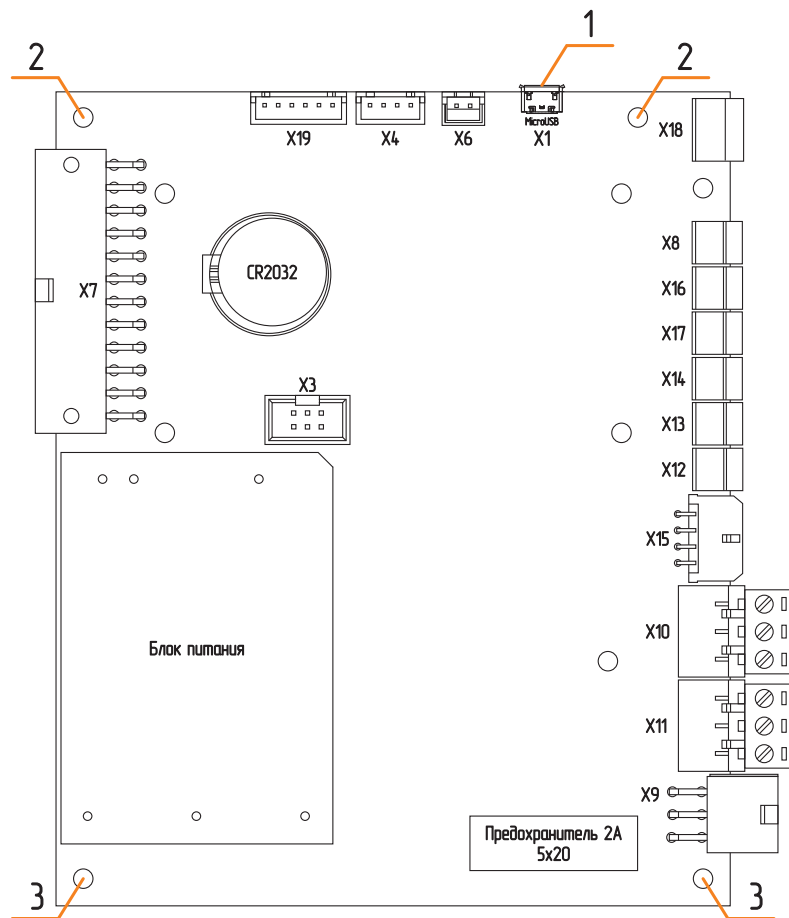
Рис.13 Плата контроллера
