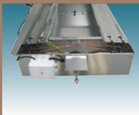
Mod. RDF350.: lato collegamento frigorifero ed elettrico. RDF350... model: pipe and electrical connection side.
