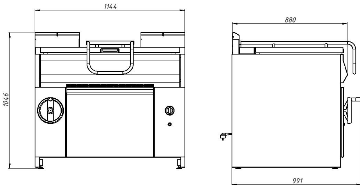
Рис.1. Габаритные размеры установки
