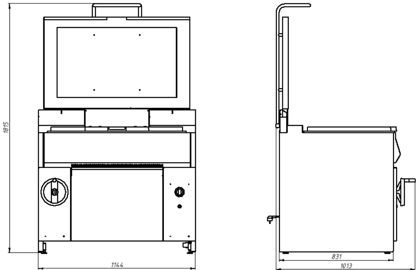
Рис.3 Вид с открытой крышкой
