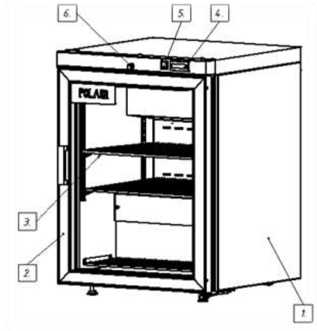
Рис. 2. Внешний вид шкафа DP102-S
