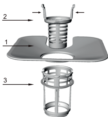
Система фильтров
