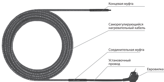
Рис. 1 - Конструкция секции нагревательной кабельной Freezstop Inside Dachа
