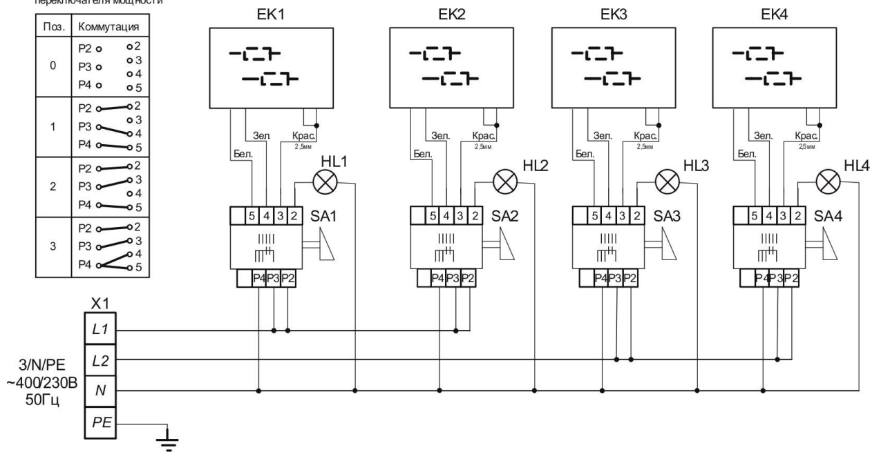
Рисунок 1 Схема электрическая для ПЭЧ-4
