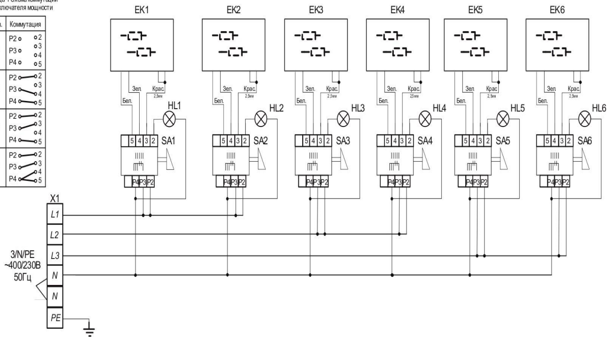
Рисунок 2 Схема электрическая для ПЭЧ-6
