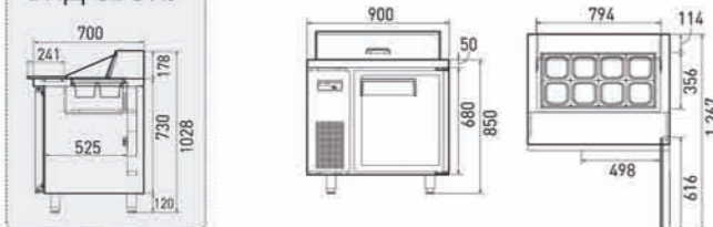
ВИД СБОКУ
