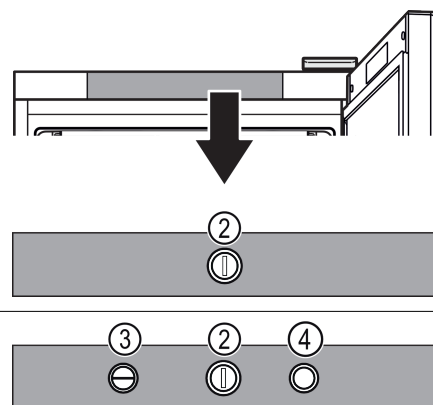
Fig. 42 (2) Регулятор температуры
