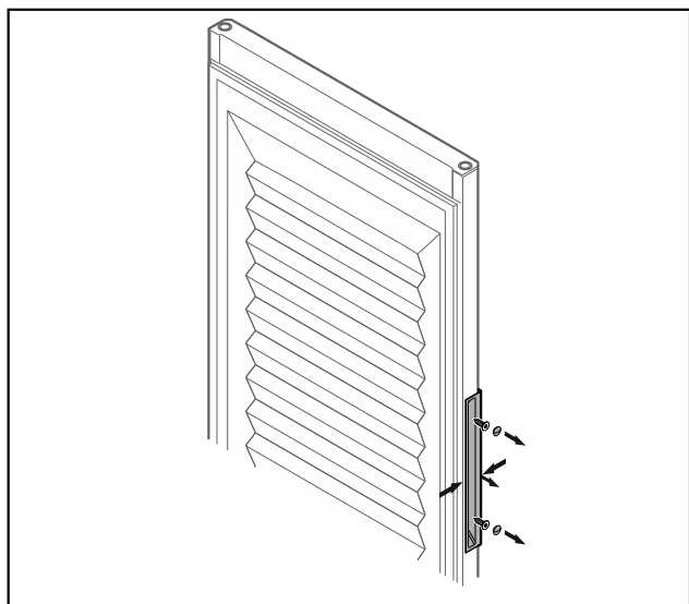
Fig. 17 Запененная дверь*
