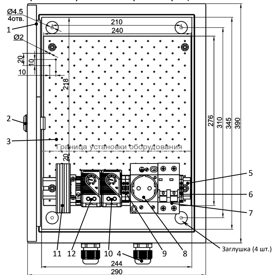
Рисунок 1 – Устройство шкафа
