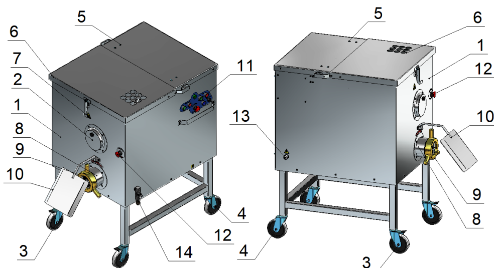
Рис. 1 Устройство мясорубки
