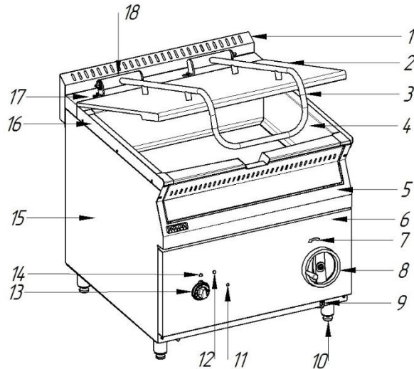
Рисунок 1 – Внешний вид сковороды электрической СЭ-40-1 МХ
