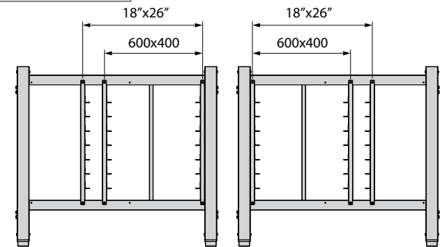
Stand XWARC-00EF-H
