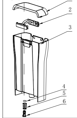
水箱组件
