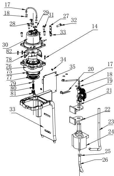
水泵支架组件
