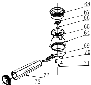
高压漏斗组件
