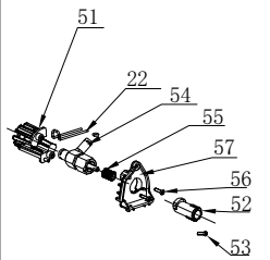
蒸汽阀体组件
