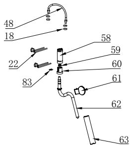
蒸汽管组件
