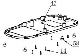
底盖组件
