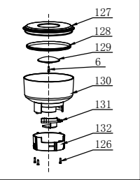
豆箱组件
