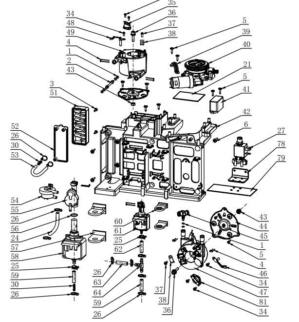
支架组件
