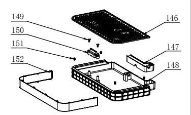
接水盘组件
