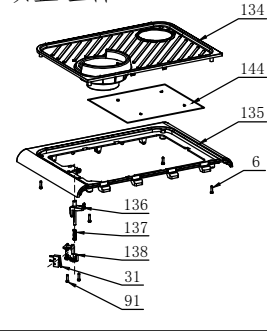
顶盖组件
