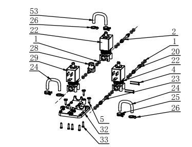
电磁阀组件
