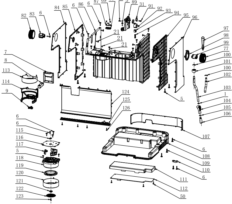
主体组件
