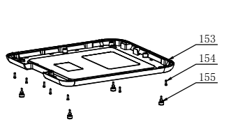
底板组件
