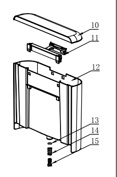
水箱组件
