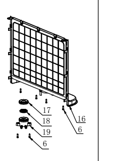
后盖组件
