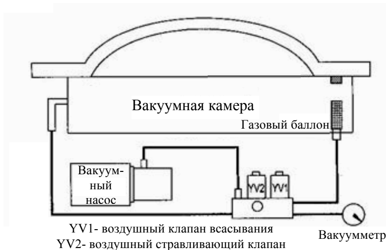
Схема вакуумного упаковщика с производительностью вакуумного насоса более 20 \text{ м}^3
