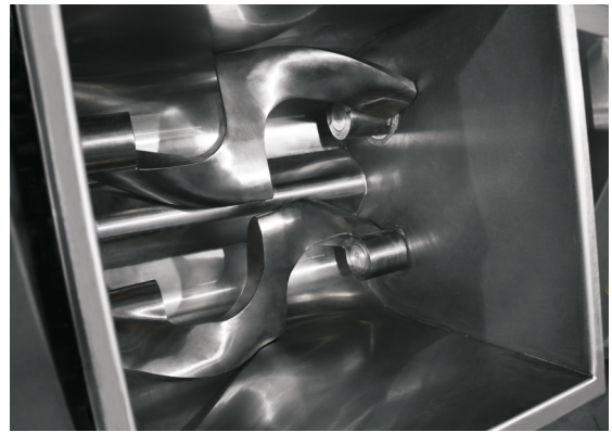
Z-образные литые нержавеющие месильные органы
